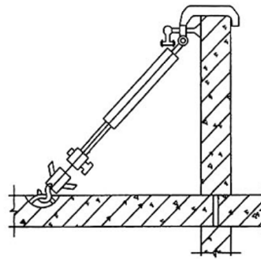
c) Thanh chống có đầu móc vít
