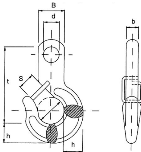
d) Móc cầu an toàn
