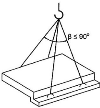
d) Chiều nghiêng cầu thang
