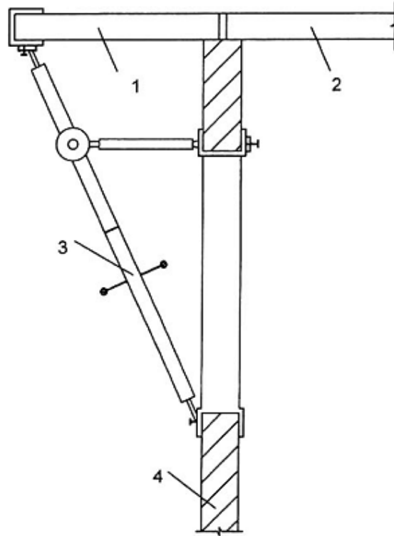
a) Bộ gá thanh chống
