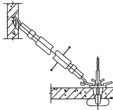
d) Thanh chống kẹp vạt năng
