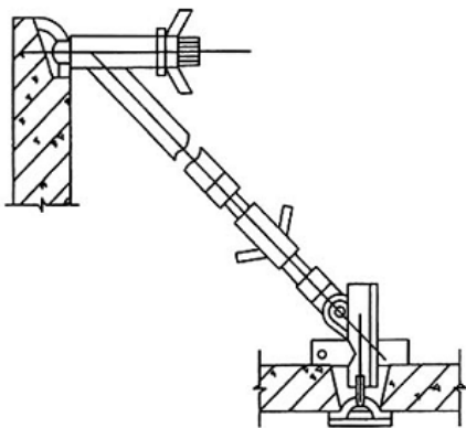
b) Thanh chống kẹp vít
