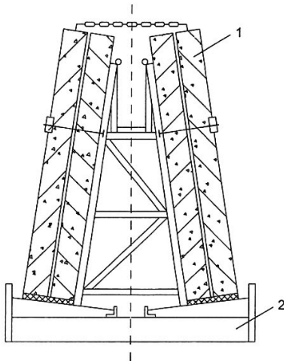
Hình 2 - Vận chuyển cấu kiện trên ca sét nghiêng
